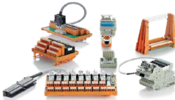
Interfaz para PLC
