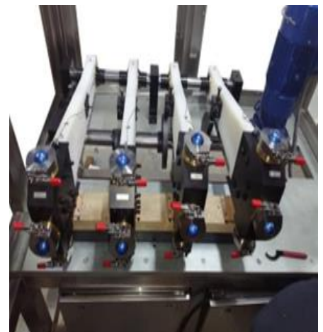
Maquinado para Pruebas de Impacto
