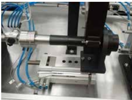
Servoprensas de hasta 1.7ton y 400mm de carrera
